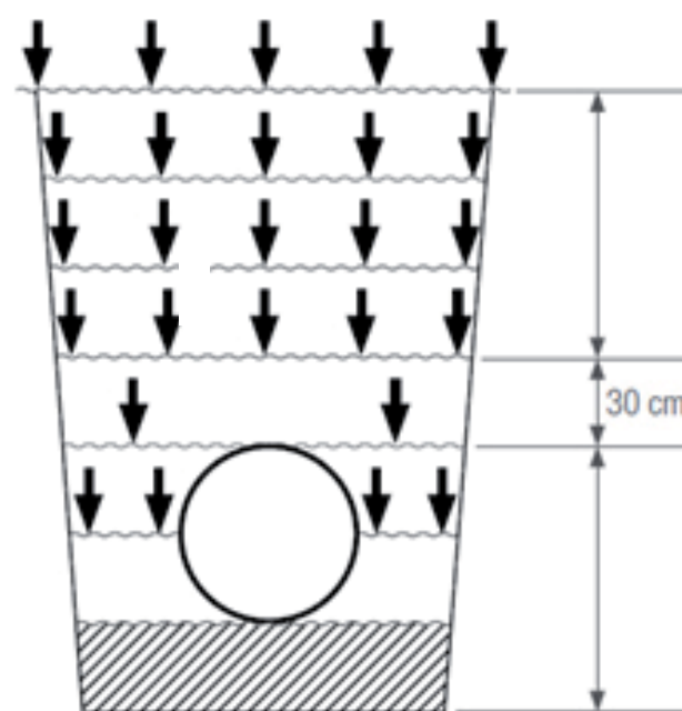
Relleno de la zanja por capas
